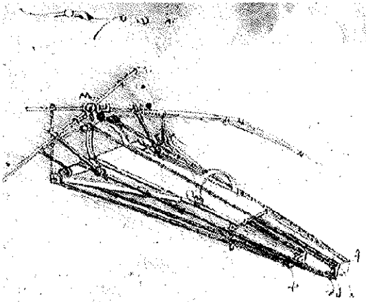
Uçuş makinası tasarımı. Sene:1488
